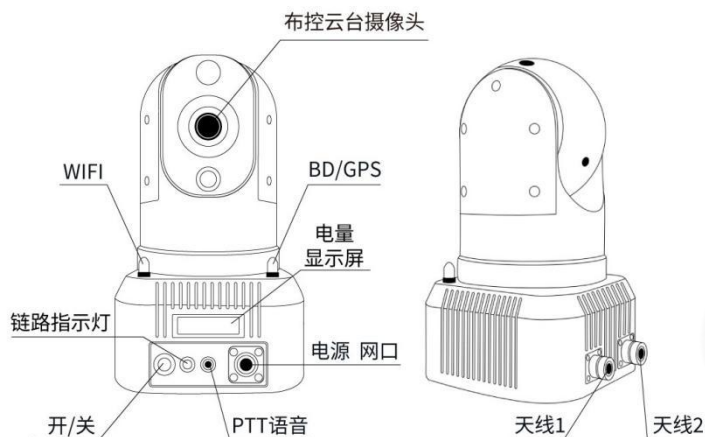
图 1 布控云台 MESH 自组网设备示意图
