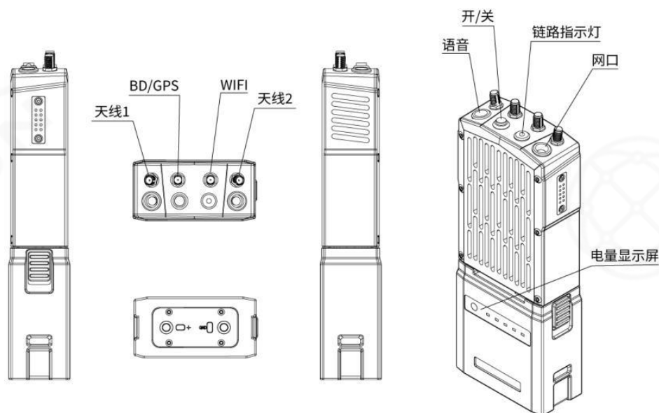
图 1 手持型 MESH 自组网设备示意图
